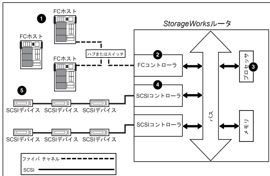
図 3: ファイバ チャンネルから SCSI へのプロトコル変換プロセス
