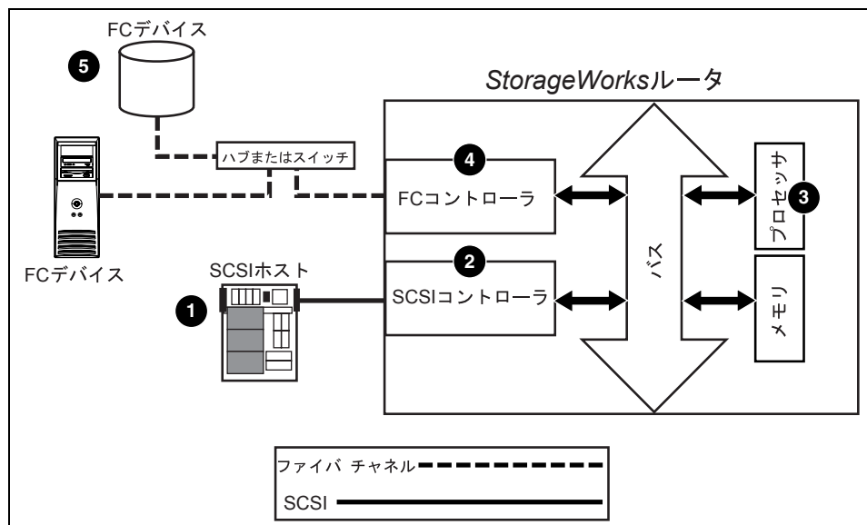
図 4: SCSI からファイバ チャンネルへのプロトコル変換プロセス
