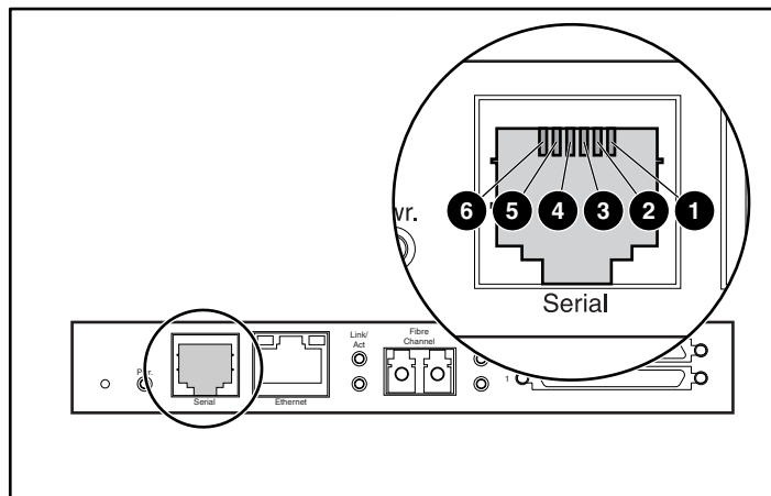
図 81: RJ-11 シリアル ピン配置
