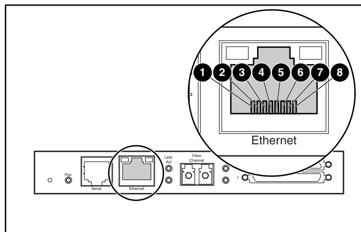
図 82: RJ-45 Ethernet ピン配置
