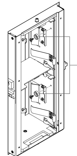
Afbeelding 4: de laadpoortnokjes bevestigen
