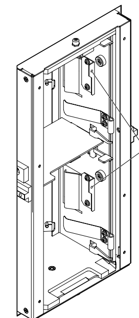
Afbeelding 5: het laadpakket installeren
